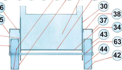
Příčný řez zadní osou (pohled ve směru jízdy)
