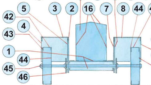
Příčný řez přední osou (pohled ve směru jízdy)
